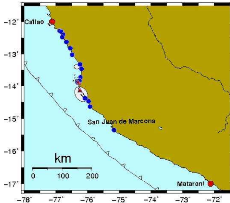
Figura 4.- Sitios donde se realizaron observaciones (círculos azules) a lo largo de la costa del Perú. Los círculos rojos muestran las ubicaciones de la estaciones en Callao y Matarani así como las dos elipses blancas representan los lugares de máximo desplazamiento en la falla.
